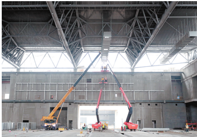
图为工人们正在对屋顶结构施工。
